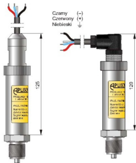
Przetwornik PC-28 z przyłączem elektrycznym typu PK Stopień ochrony obudowy IP-67 Przyłącze elektryczne kablowe, połączenie z atmosferą przez kapilarę znajdującą się w kablu, długość kabla 3 m (inna długość kabla – na zamówienie)
