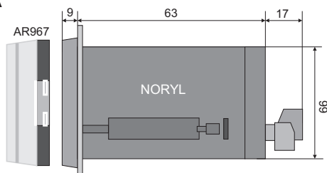
WIDOK OD STRONY UCHWYTU MOCUJĄCEGO
